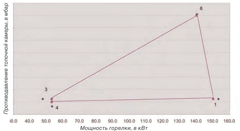
Рабочее поле горелки НРМ 4, для природного газа G20, G25
