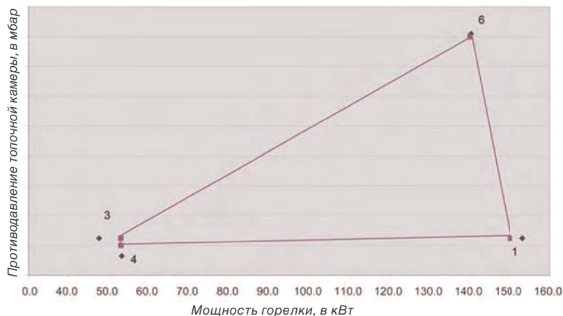
Рабочее поле горелки НРМ 2, для природного газа G20
