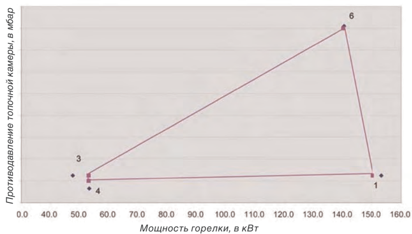
Рабочее поле горелки НРМ 3, для природного газа G20, G25
